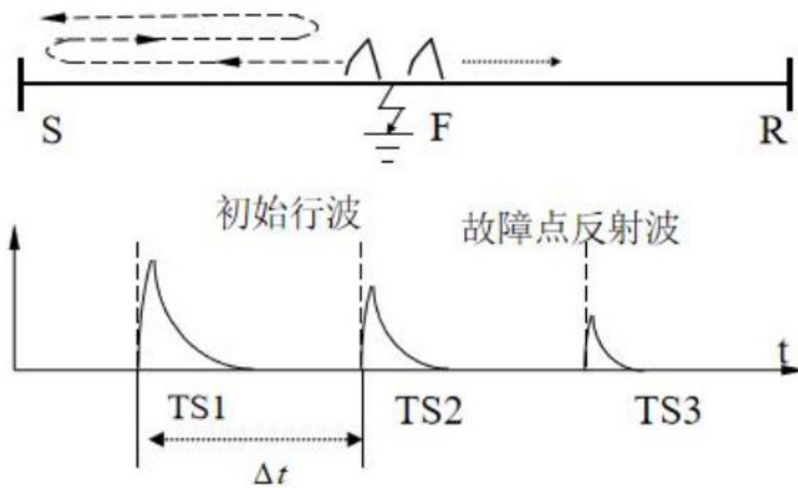
单端测距
